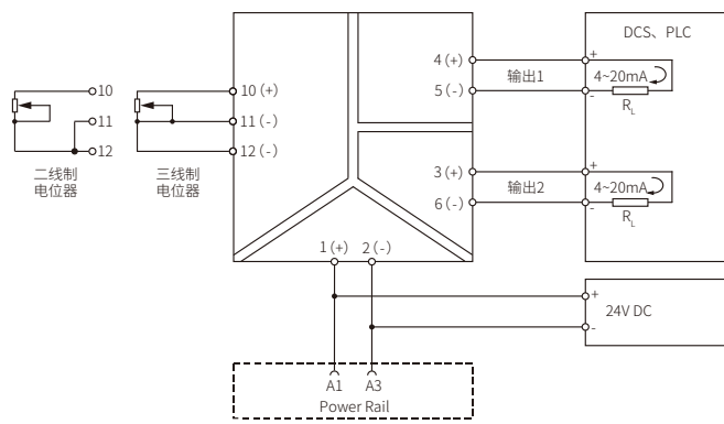
CZ3576.R (CZ3575输出部分仅包含输出1)
