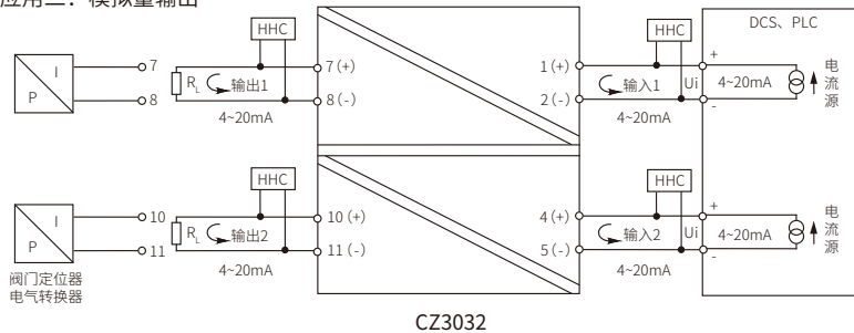
应用二：模拟量输出
