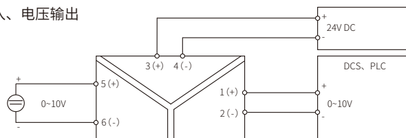
应用四：电压输入、电压输出
