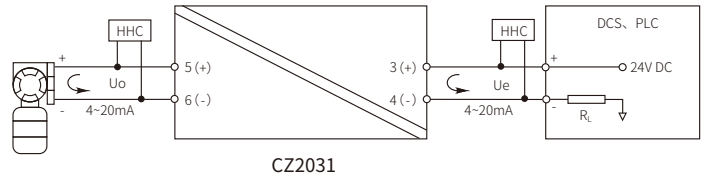
应用一：模拟量输入
