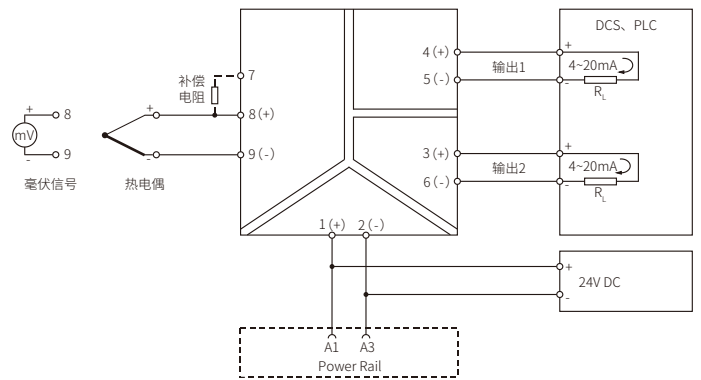
CZ3574(CZ3572输出部分仅包含输出1)
